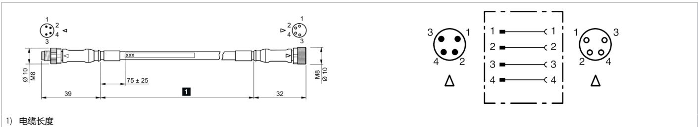
1) 电缆长度
