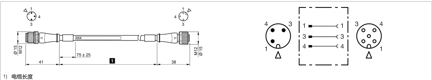
1) 电缆长度
