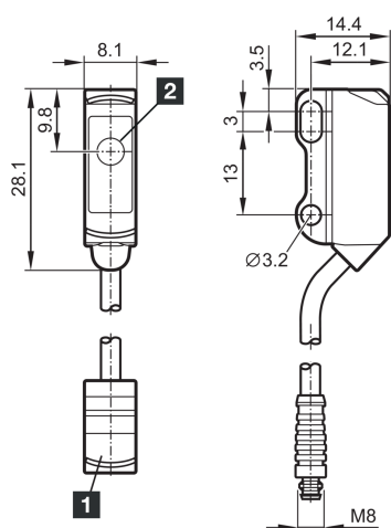
2) 发射器
