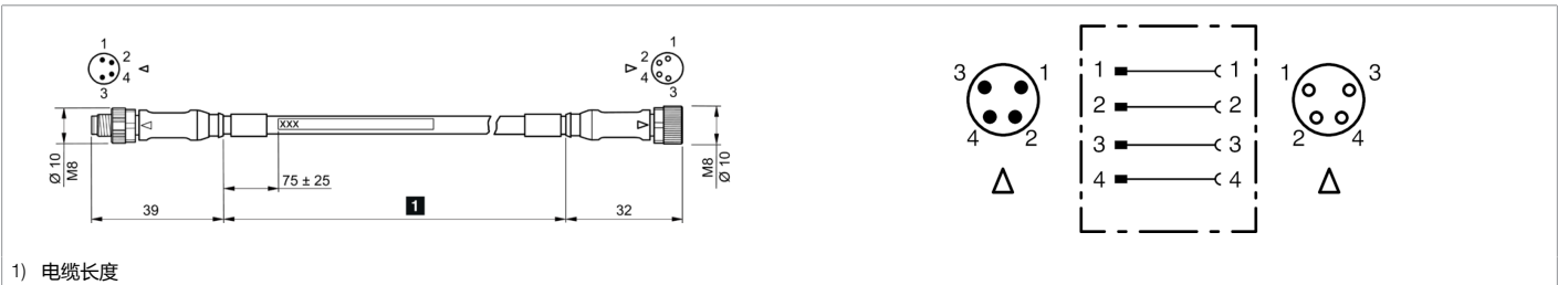
1) 电缆长度
