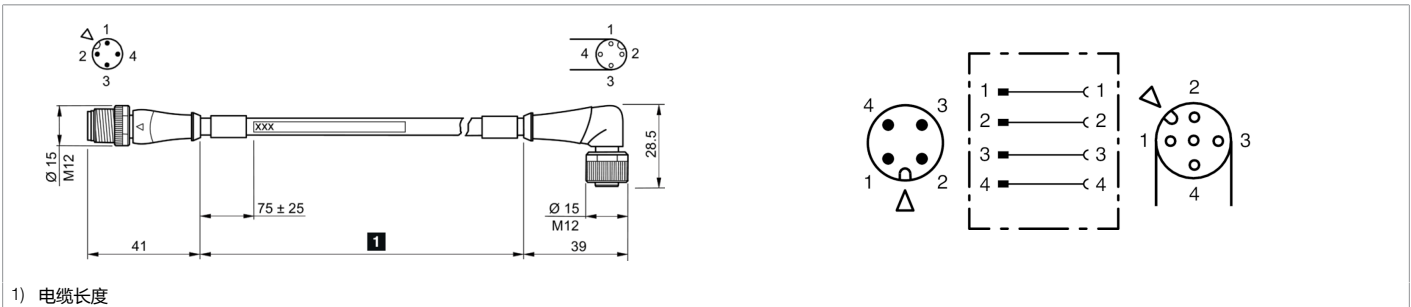
1) 电缆长度
