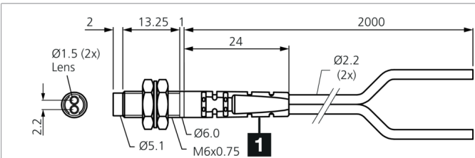
1) 电缆保护套
