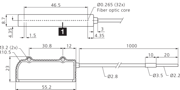
1) 光纤线芯
