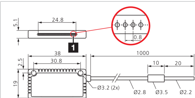
1) 光纤线芯
