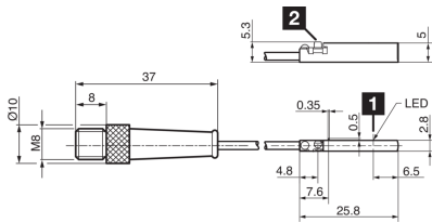
1) 感应面 2) 固定偏心件 BK: 黑色 BN: 棕色 BU: 蓝色
