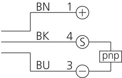
BN: 棕色
