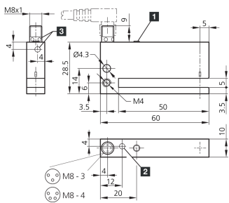
1) 示教按钮 2) 工作 LED 3) 状态 LED (黄色)
