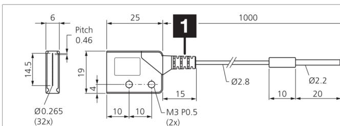
1) Cable grommet
