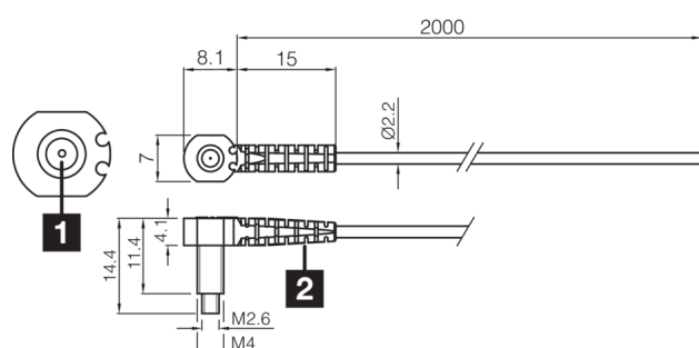
2) Cable grommet
